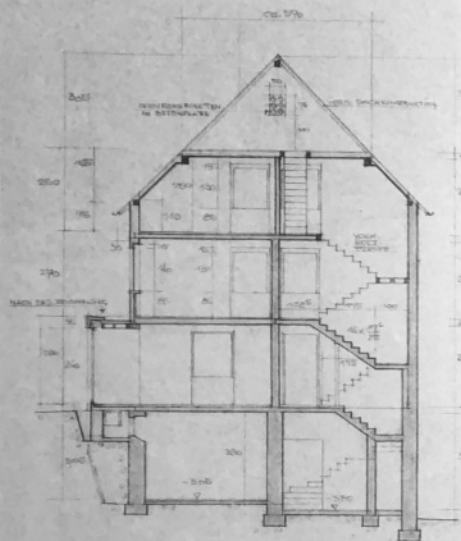
SCHNITT A-B
