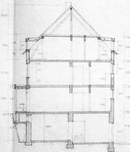
SCHNITT C-D
