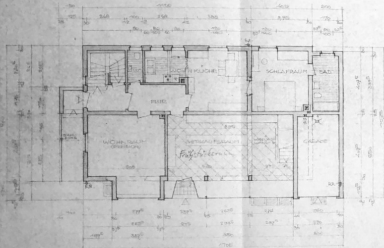
ERDGESCHOSS
